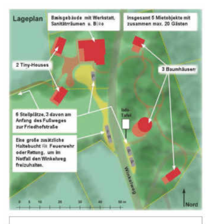
Lageplan Baumhausanlage
